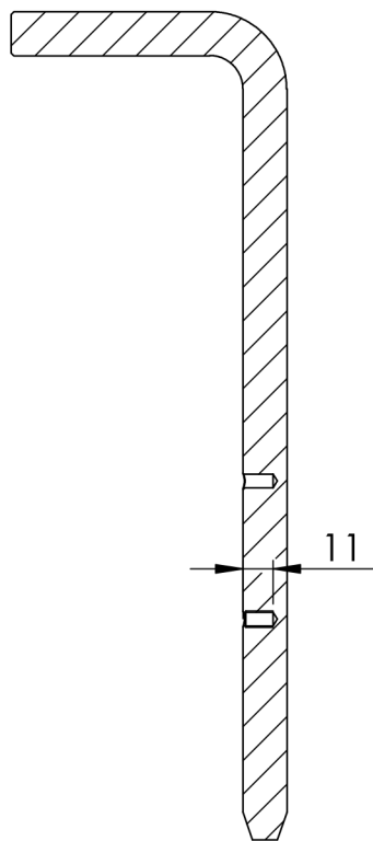
SCHNITT B-B
